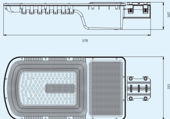
产品尺寸图 (尺寸单位: mm)
